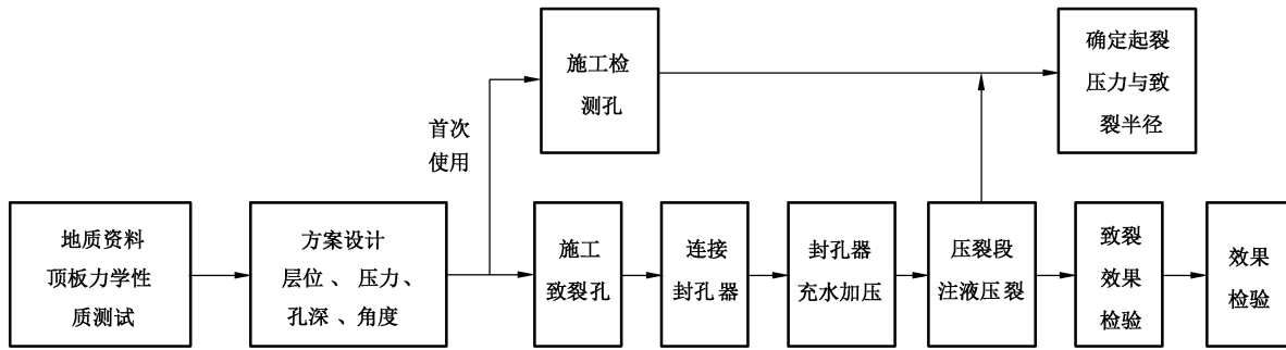
图 1 直接水压致裂施工工艺流程图
