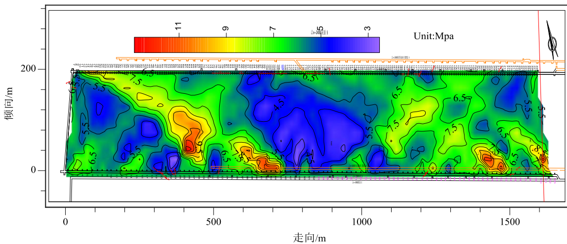
弹性波 CT 探测结果样例
