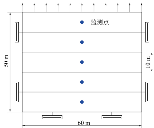
图 3 UDEC 数值模型
