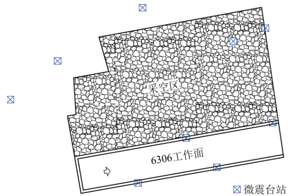
图 9 工作面及微震台站布置
