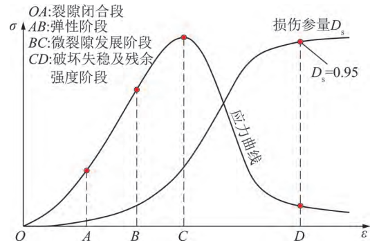
图10 煤岩体受载过程中全应力应变及损伤参量变化
