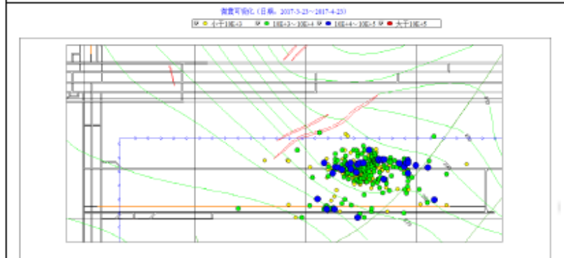
震源分布图
