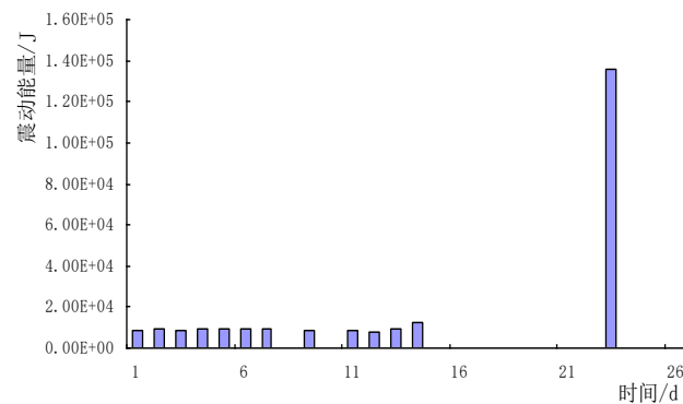
频繁-平静型微震活动
